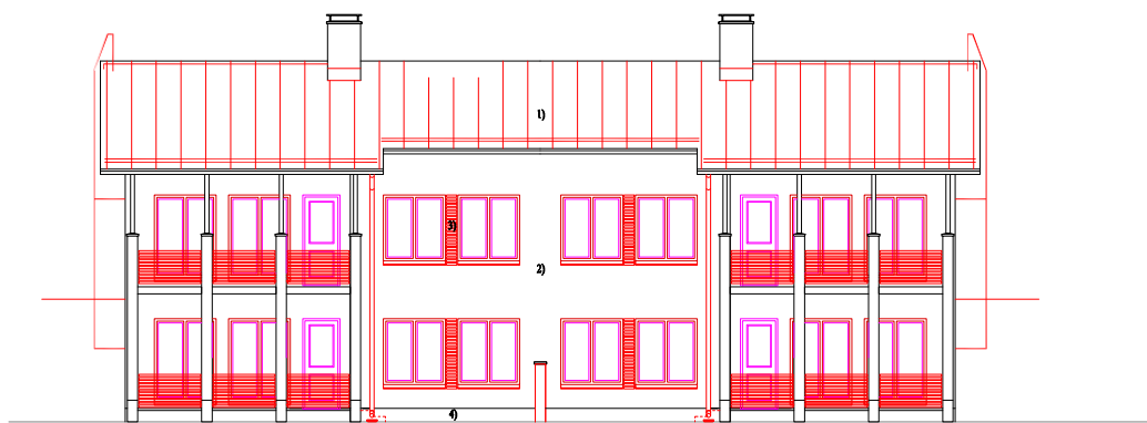
JULKISIVU (TAKAPIHALLE)
