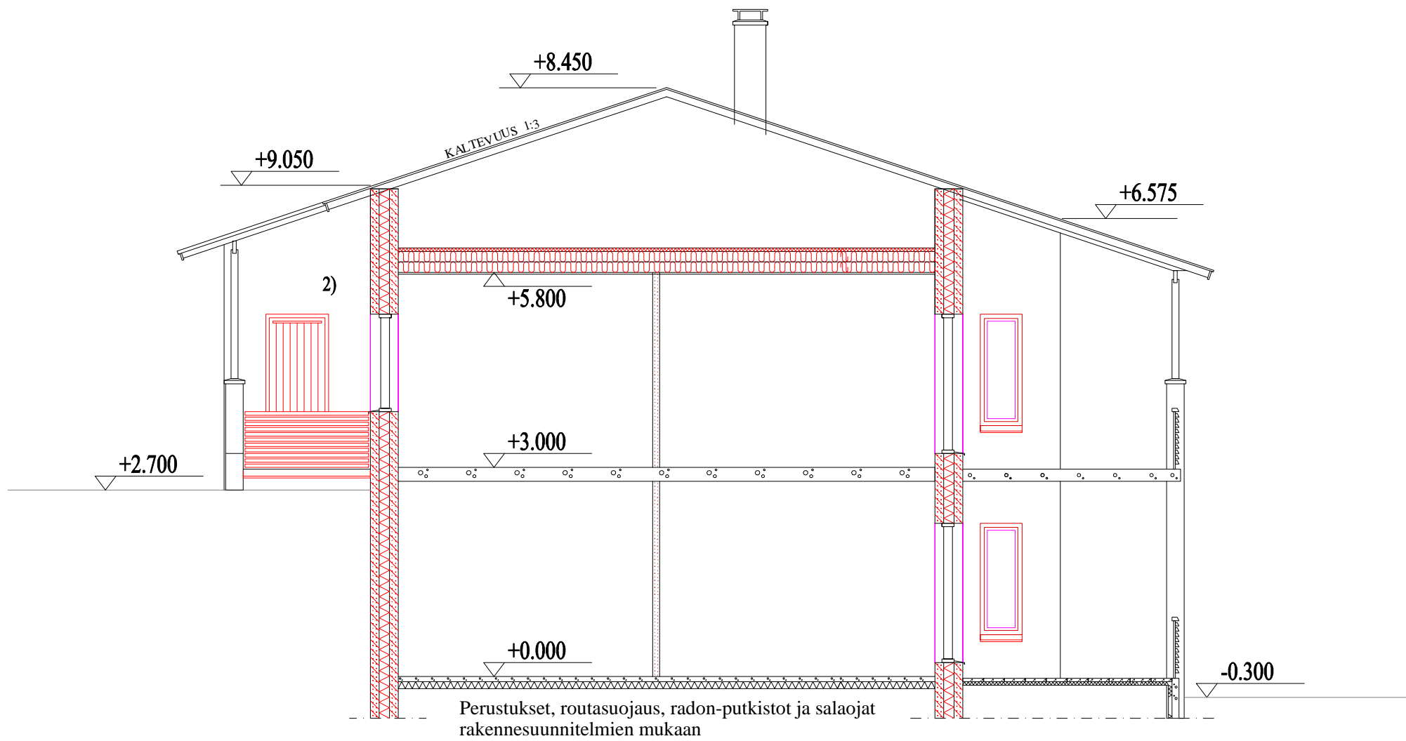
LEIKKAUS A-A
